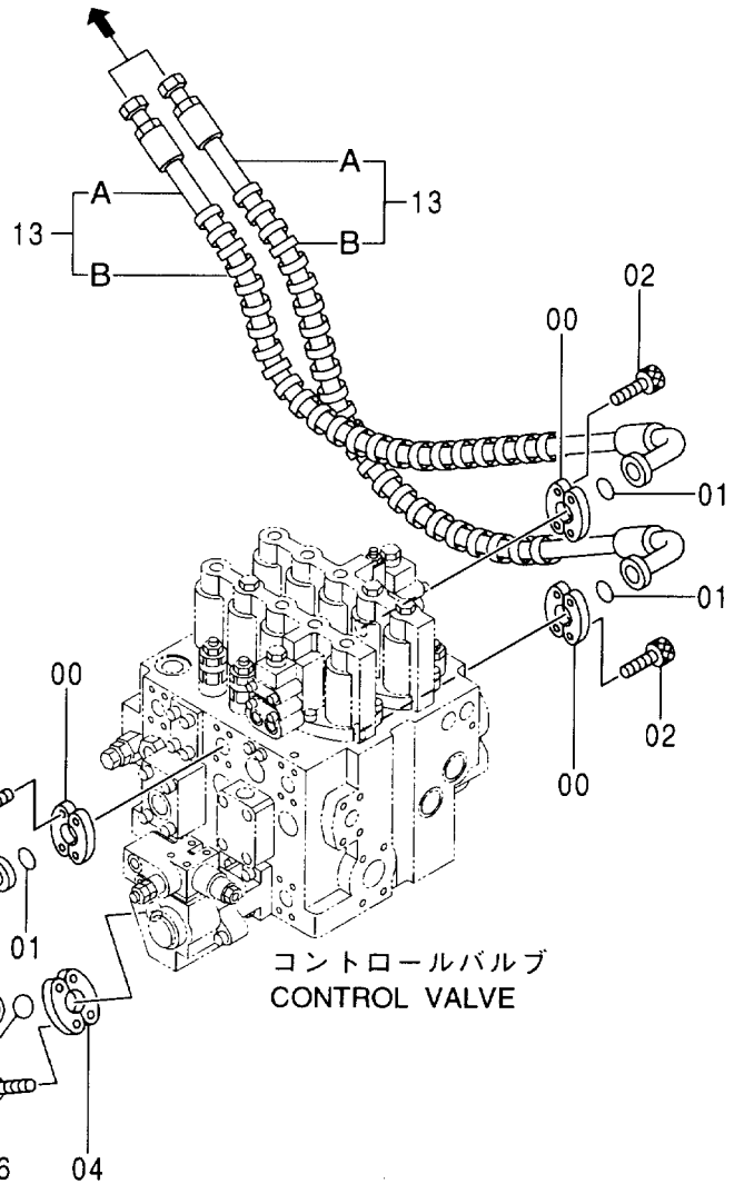
フロント配管 FRONT PIPING
