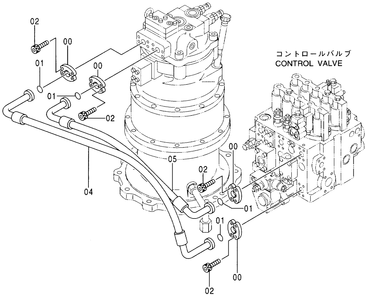
旋回装置 SWING DEVICE
