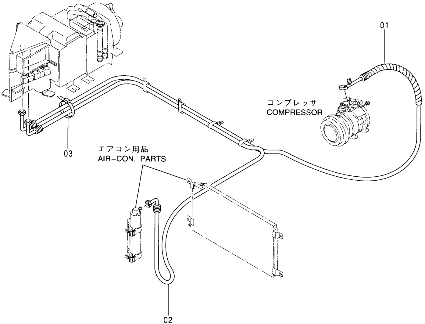
エアコンユニット AIR-CON. UNIT
