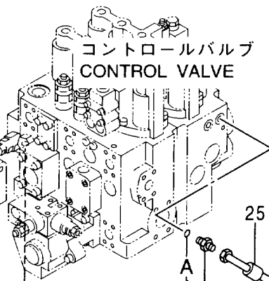
ソレノイドバルブ SOLENOID VALVE
