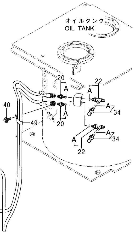
コントロールバルブ CONTROL VALVE
