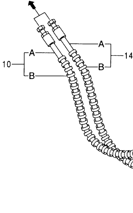
フロント配管 FRONT PIPING
