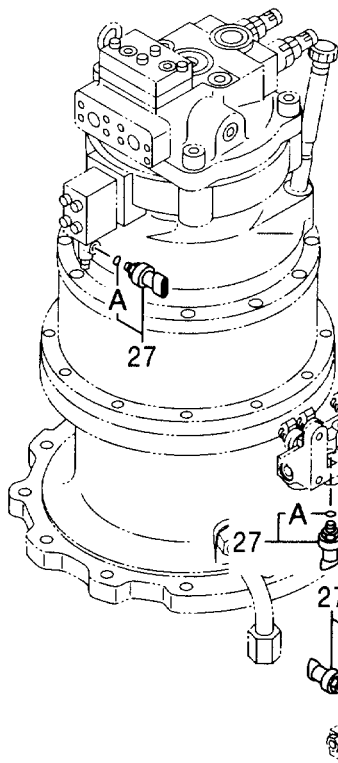
パイロット配管 (4) PILOT PIPING (4)
