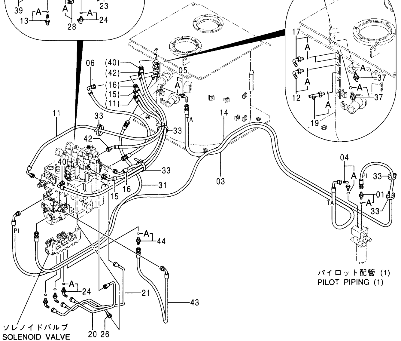
パイロット配管 (5-1) PILOT PIPING (5-1)
